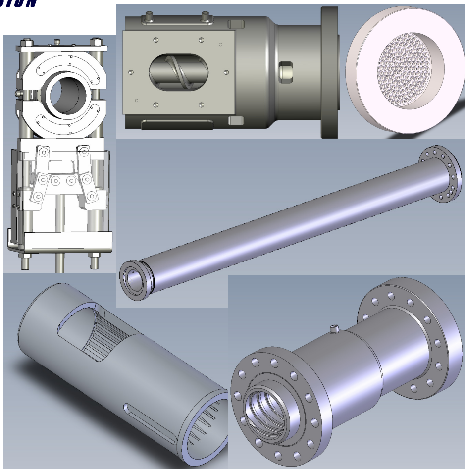
Composants mécaniques pour extrudeuses
